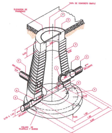
DETALLE DE POZO DE VISITA
