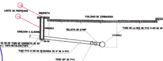
DETALLE DE CONEXIÓN DE DESCARGAS
