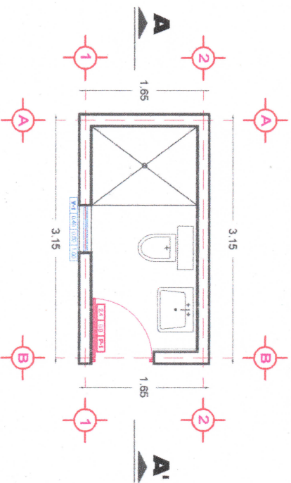
PLANTA ARQUITECTONICA TIPO
