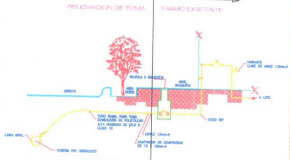
DETALLE "TIPO" TOMA DOMICILIARIA DE VIVIENDA SIN SERVIDOR DETALLES CONSTRUCTIVOS
