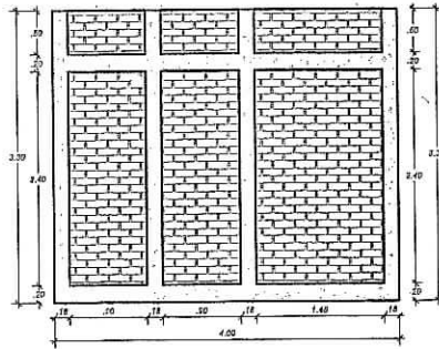
FACHADA LATERAL TIPO
