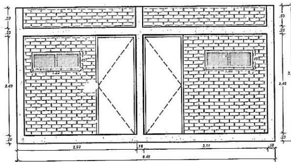
FACHADA FRONTAL TIPO
