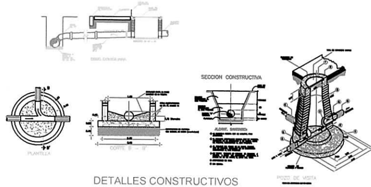
DETALLES CONSTRUCTIVOS
